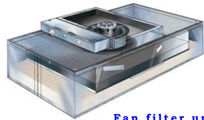
Fan filter unit
